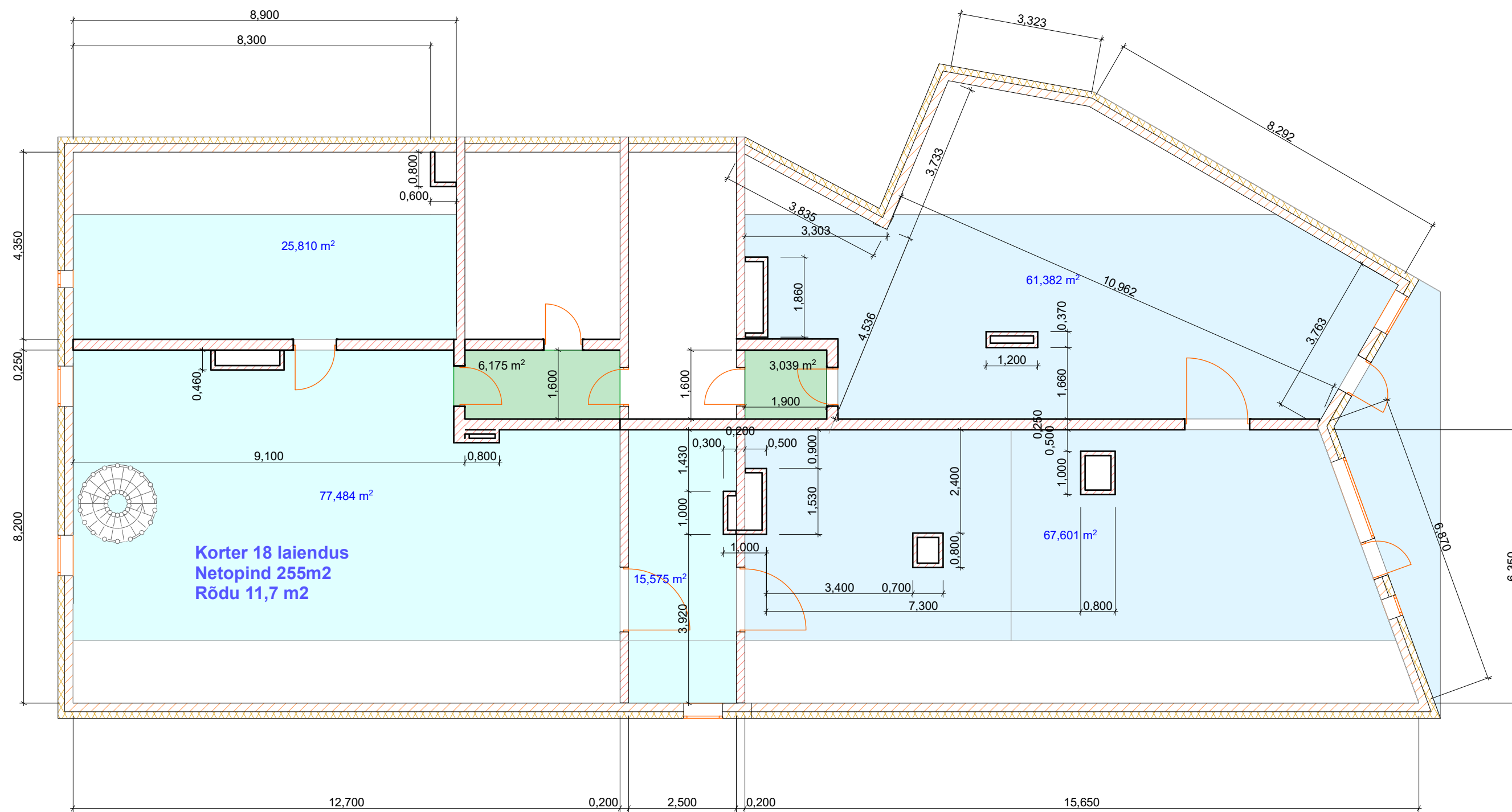
Pööningukorruse laiendus 1:100
