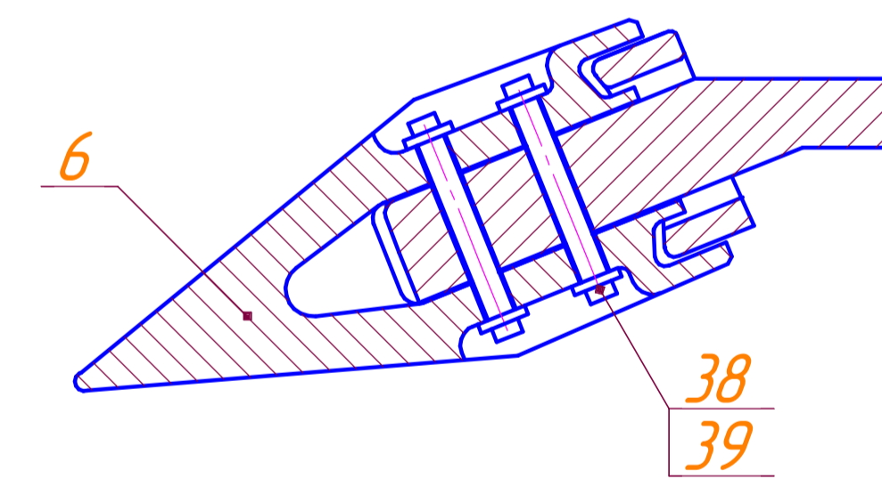
Установка зубьев (1:10)
