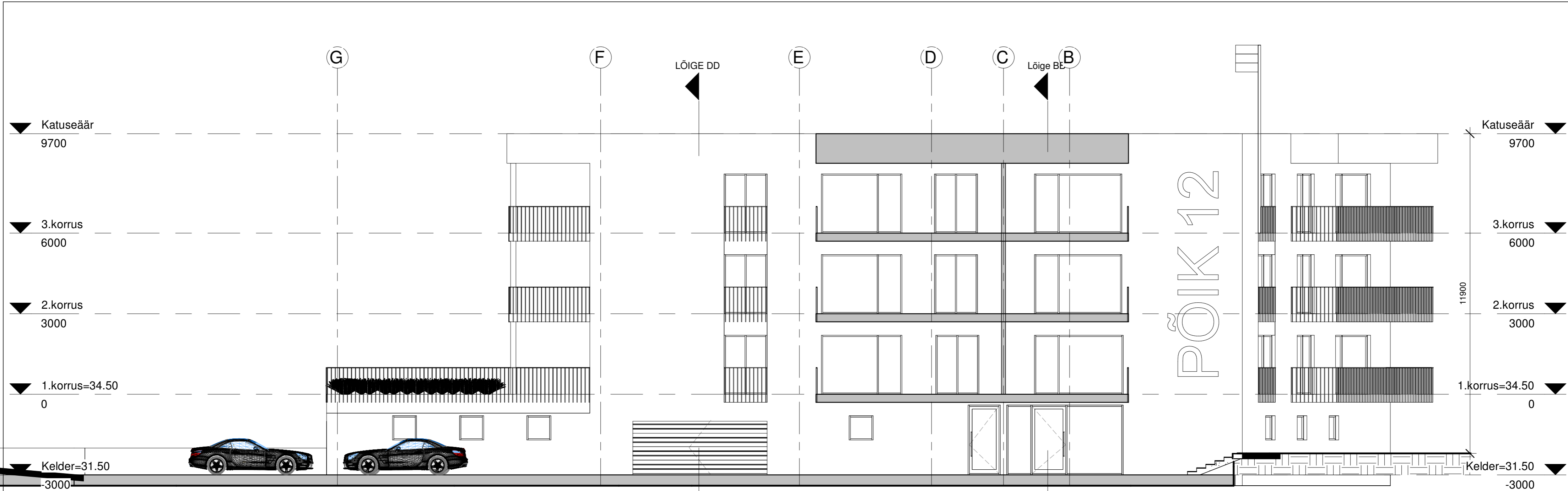
1 Lõige CC 1 : 100
