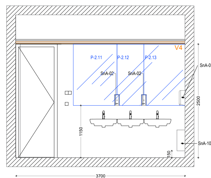
Lõige 1-1 L112
