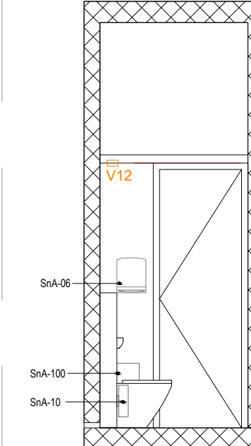
Lõige 1-1 L333
