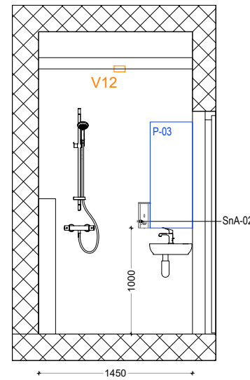
Lõige 3-3 L203
