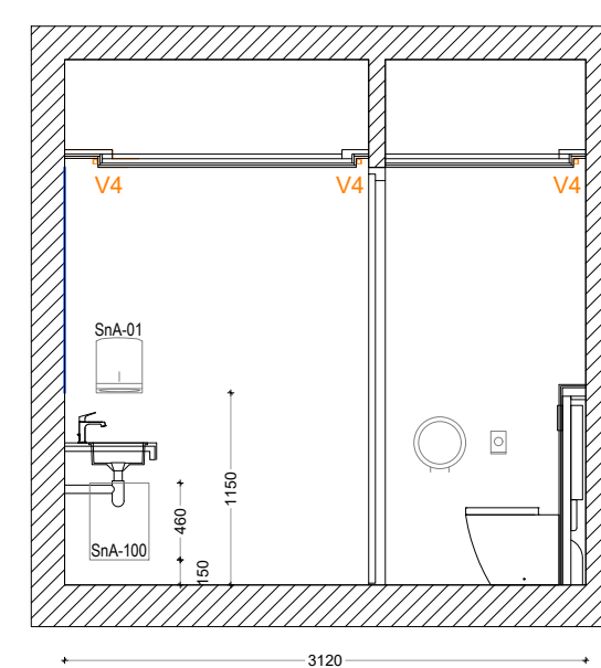
Lõige 2-2 L112
