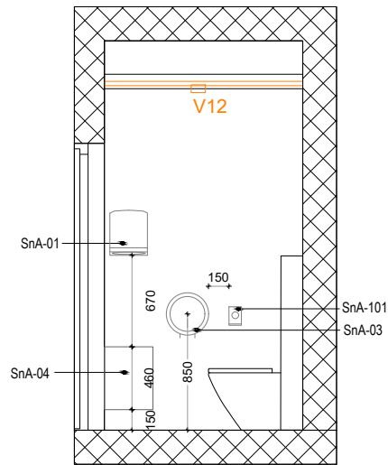
Lõige 2-2 L204
