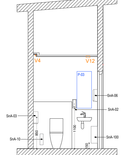
Lõige 2-2 L333
