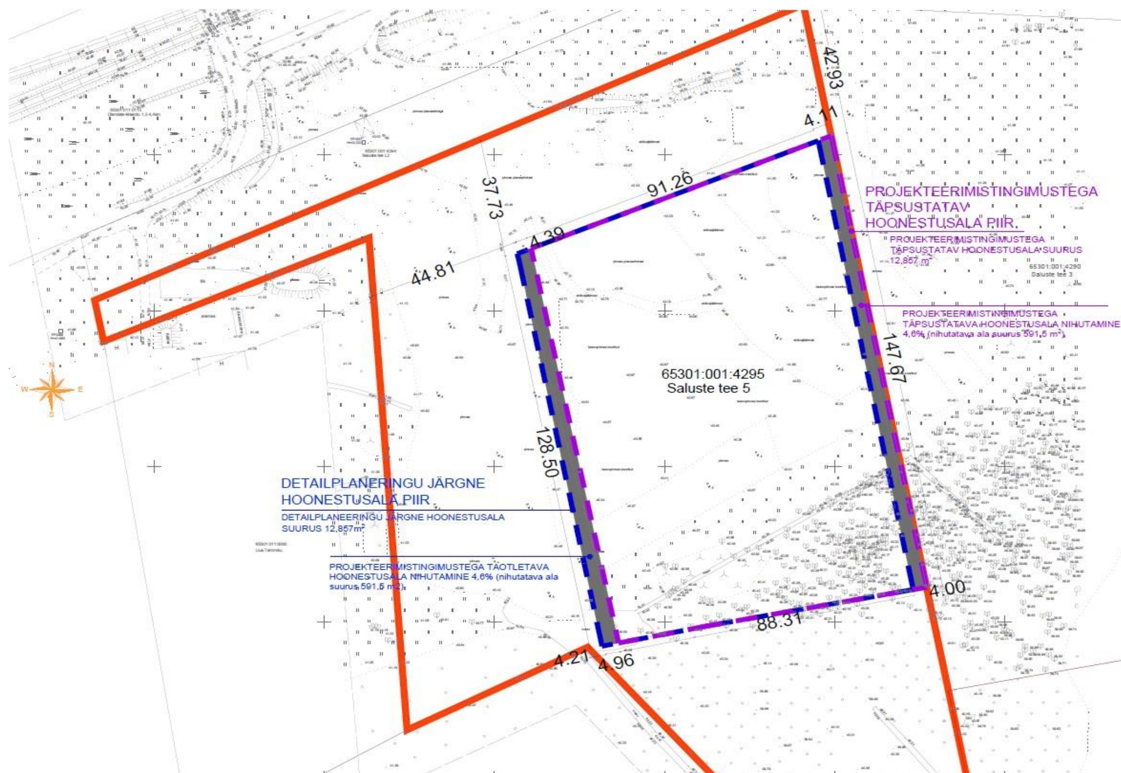
Skeem 1. Soodevahe küla Tammiku 1 kinnistu ja lähiala detailplaneeringu põhijoonise krundipositsiooni 1 hoonestusala nihutamine 4,59%, s.o ca 4,1 m võrra idapoolsele kinnistupiirile lähemale.
