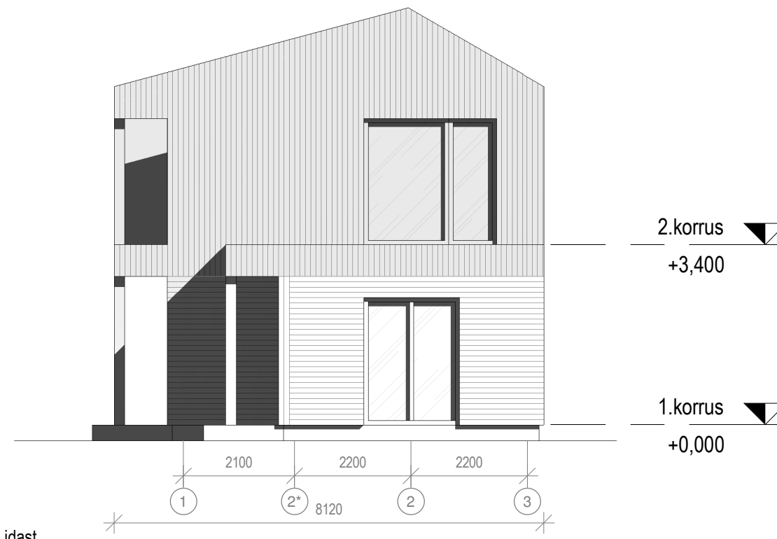
Vaade idast 1 : 100
