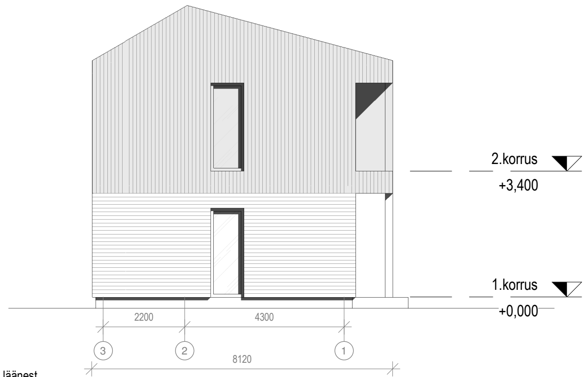
Vaade läänest 1 : 100
