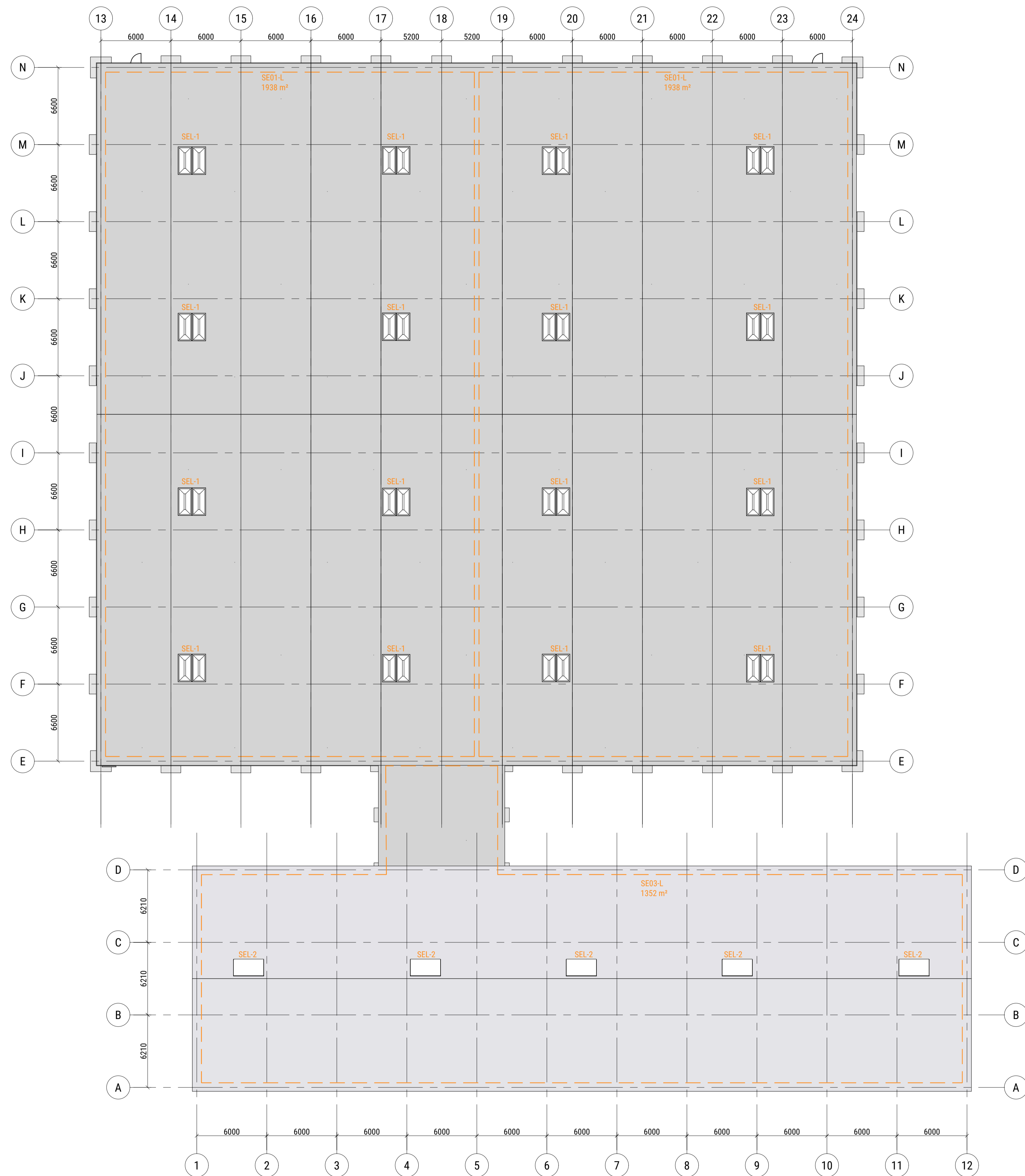
KATUSEPLAAN 1:200
