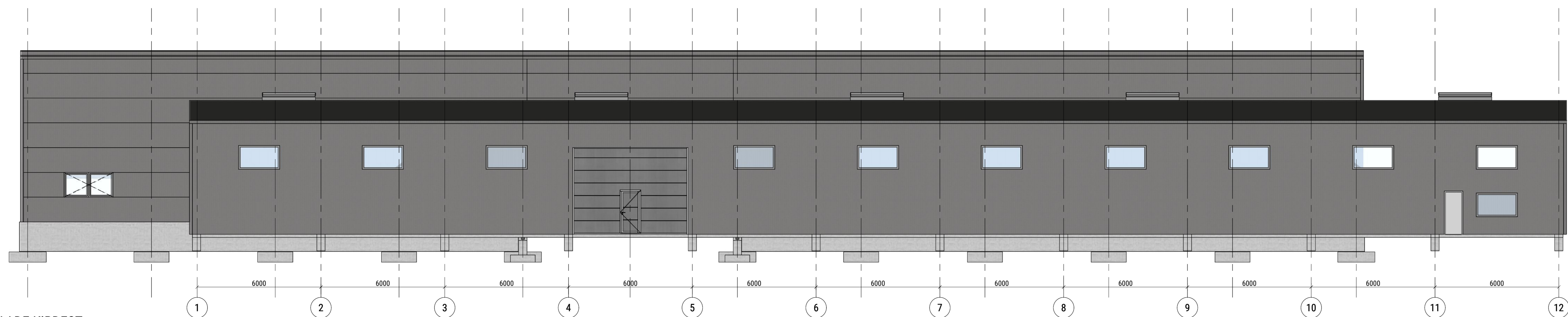
VAADE KIRDEST 1:100
